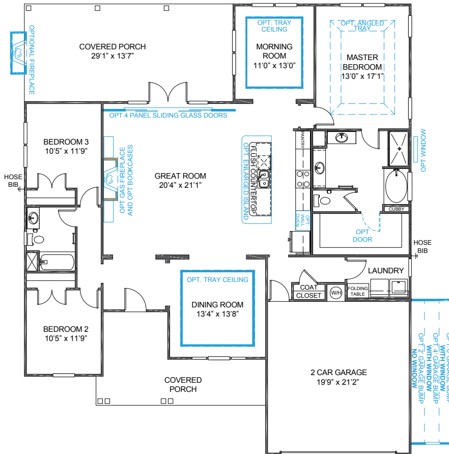
PLAN 2230
